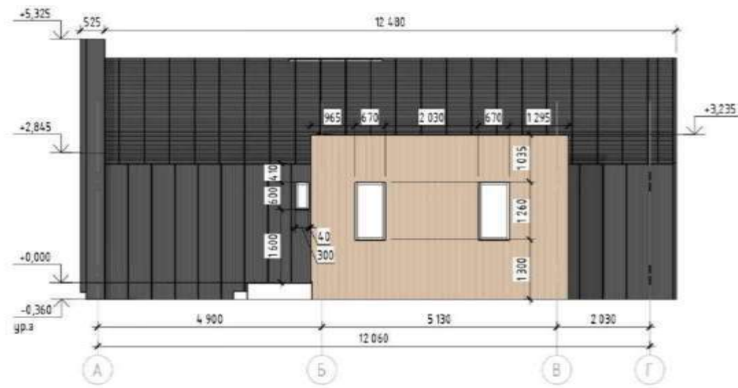
М 1:80 | Фасад А-Г
