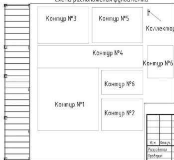
Схема расположения фундамента
