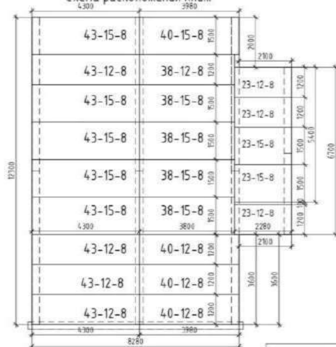
Схема расположения плит
