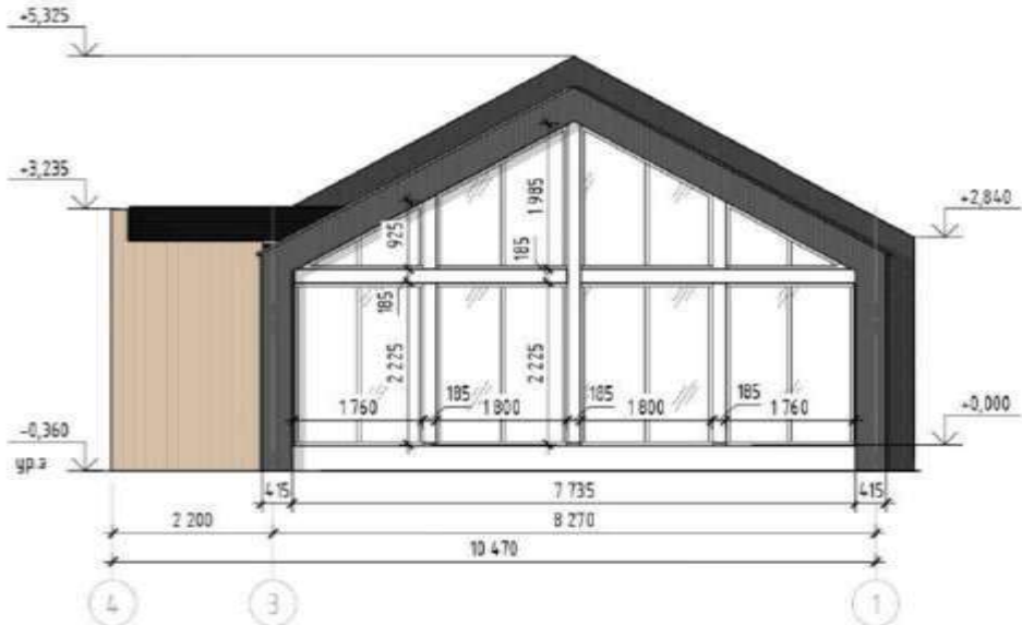
М 1:80 | Фасад 4-1
