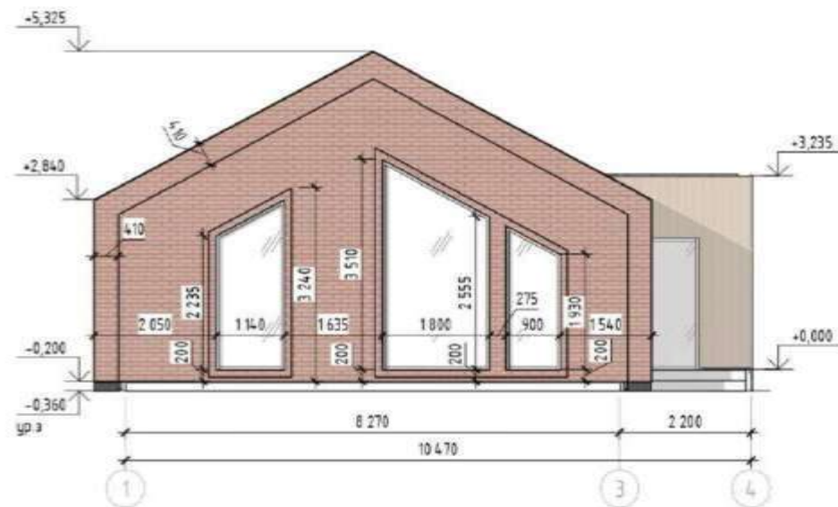
М 1:80 | Фасад 1-4
