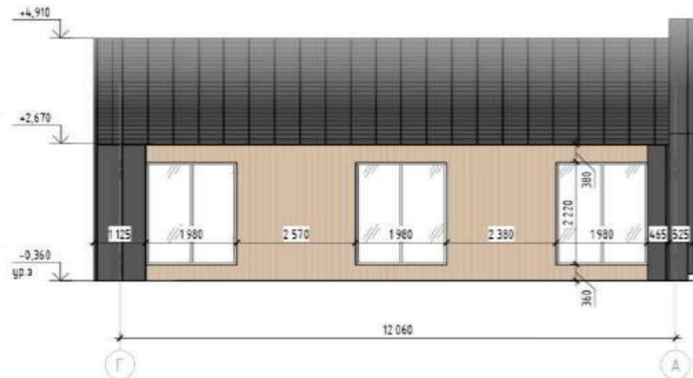
М 1:80 | Фасад Г-А
