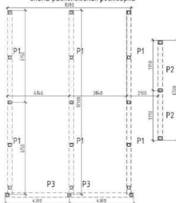
Схема расположения ростверка
