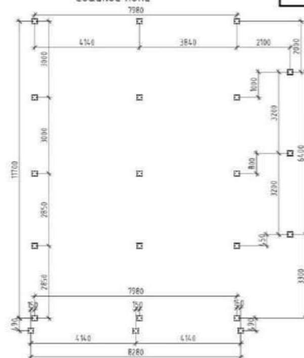
Свайное поле
